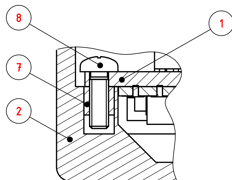
DETALLE B (4 : 1)
